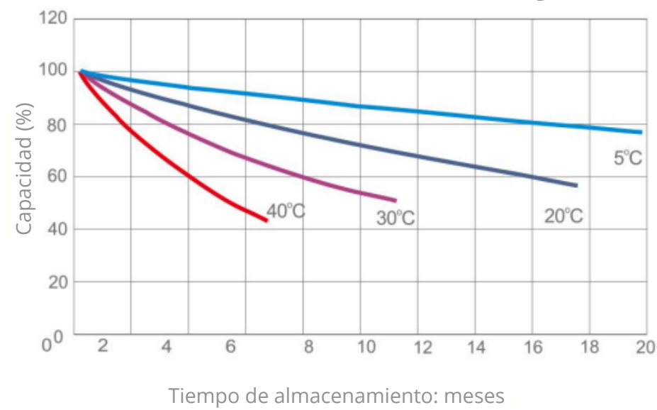
Características de auto descarga
